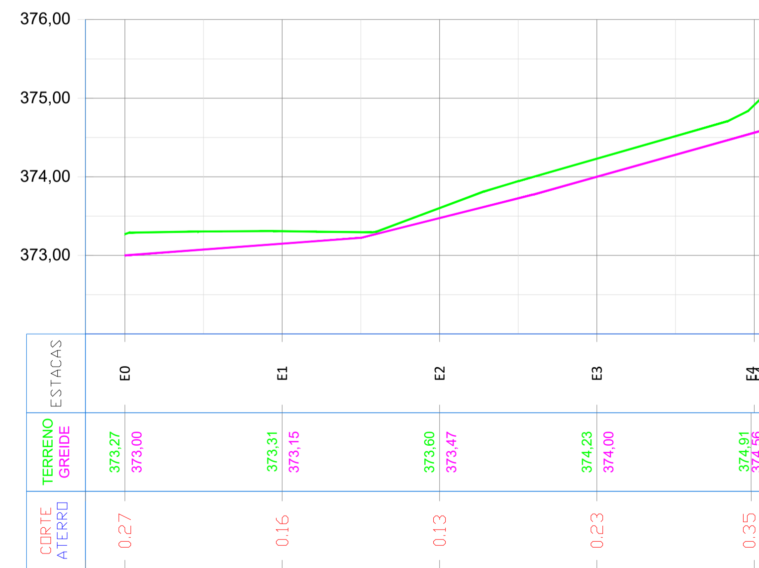
Rua B Exagero Vert. 10 Escala Vert 1:100
