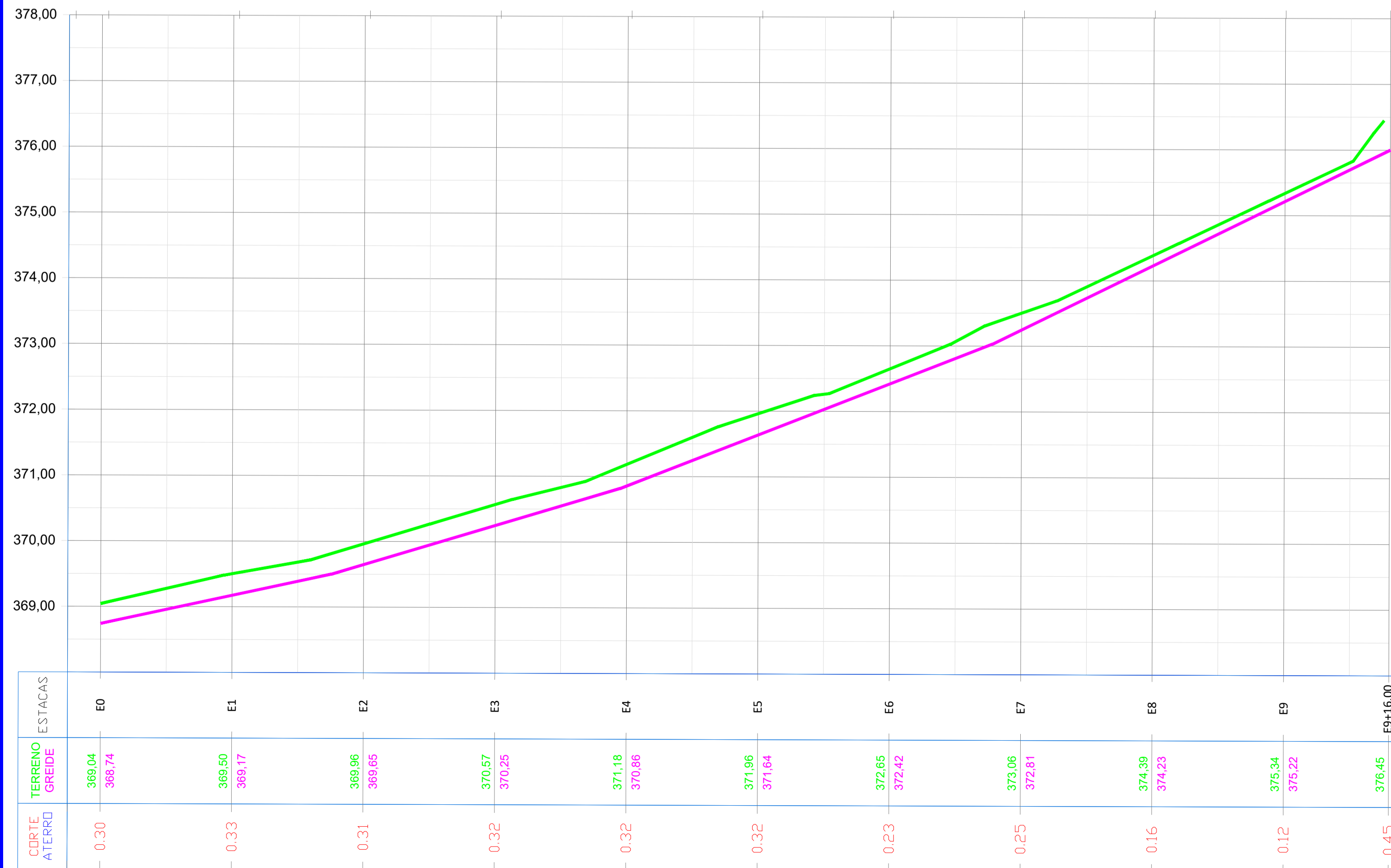
RUA A Exagero Vert. 10 Escala Vert 1:100
