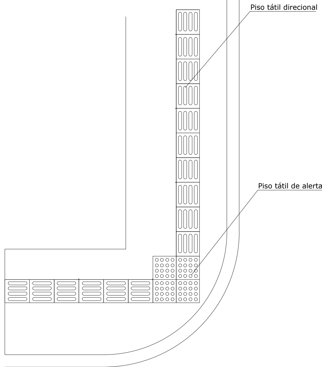
PLANTA BAIXA - DETALHE PISO TÁTIL S/ ESCALA
